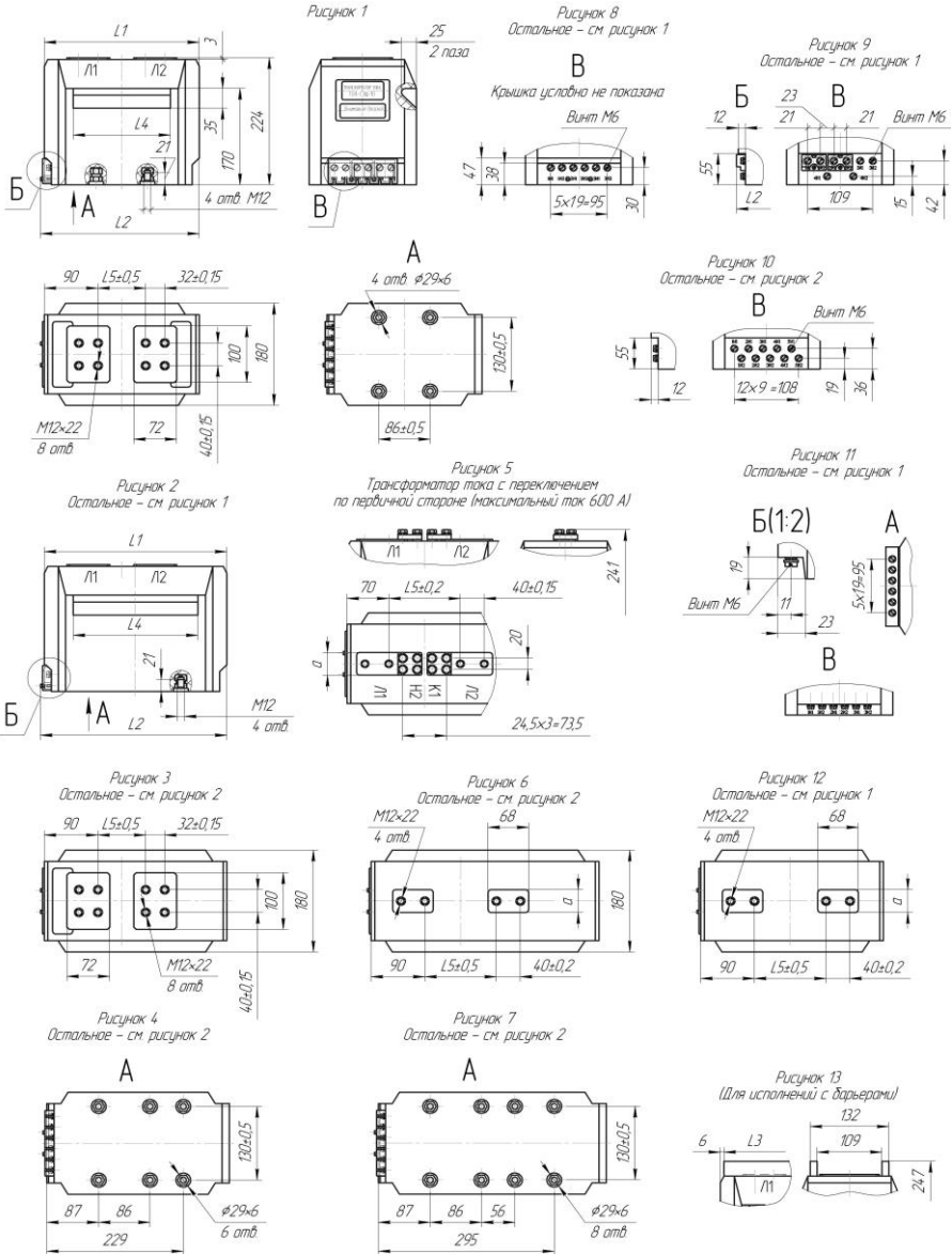
Рисунок 5 Габаритные, установочные и присоединительные размеры трансформаторов тока ТОЛ-СЭЩ-10 исполнений 11÷14-1, 21÷24-1, 31÷34-1, 41÷44-1, 51÷54-1, 61÷64-1, 71÷74-1, 81÷84-1
