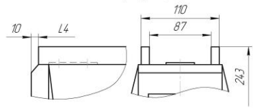
Рисунок 3 Трансформатор тока с дьярьерами Остальное см рисунки 1, 2, 4
