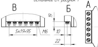
Рисунок 3 Остальное см. рисунок 1
