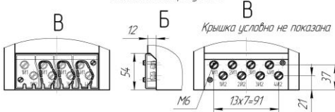
Рисунок 3 Остальное см. рисунок 1
