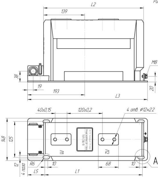
Рисунок 1 Габаритные, установочные и присоединительные размеры трансформаторов тока ТОЛ-СЭЦ-10 исполнений 01÷09
