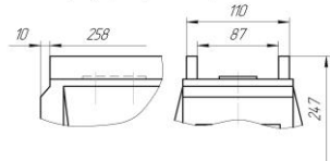
Рисунок 3 (Остальное – см рисунок 1)
