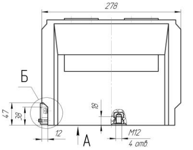
Рисунок 2 Габаритные, установочные и присоединительные размеры трансформаторов тока ТОЛ-СЭЩ-10 исполнений 11÷14, 21÷24
