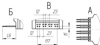
Рисунок 15 Остальное – см. рисунок 1
