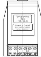
Рисунок 4 Остальное см. рисунок 1
