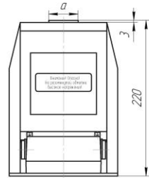
Рисунок 1 Габаритные, установочные и присоединительные размеры трансформаторов тока ТОЛ-СЭЦ-10 исполнений 01÷09
