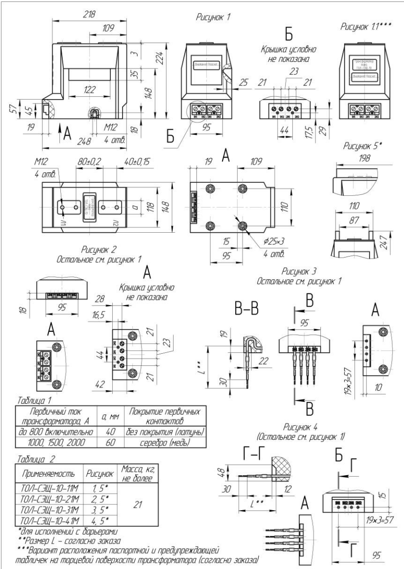
Рисунок 6 Габаритные, установочные и присоединительные размеры трансформаторов тока ТОЛ-СЭЦ-10 исполнений 11М, 21М, 31М, 41М
