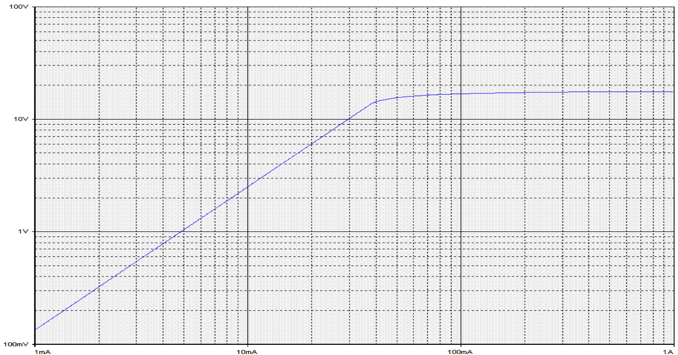
ВАХ вторичной обмотки для измерения с КТ 0,5; 0,5S, номинальной нагрузкой 10 \text{ В} \cdot \text{А} и K_{\text{БНОМ}}=10 трансформаторов с первичным током 1500 А. Сопротивление обмотки постоянному току – 0,16 Ом.
