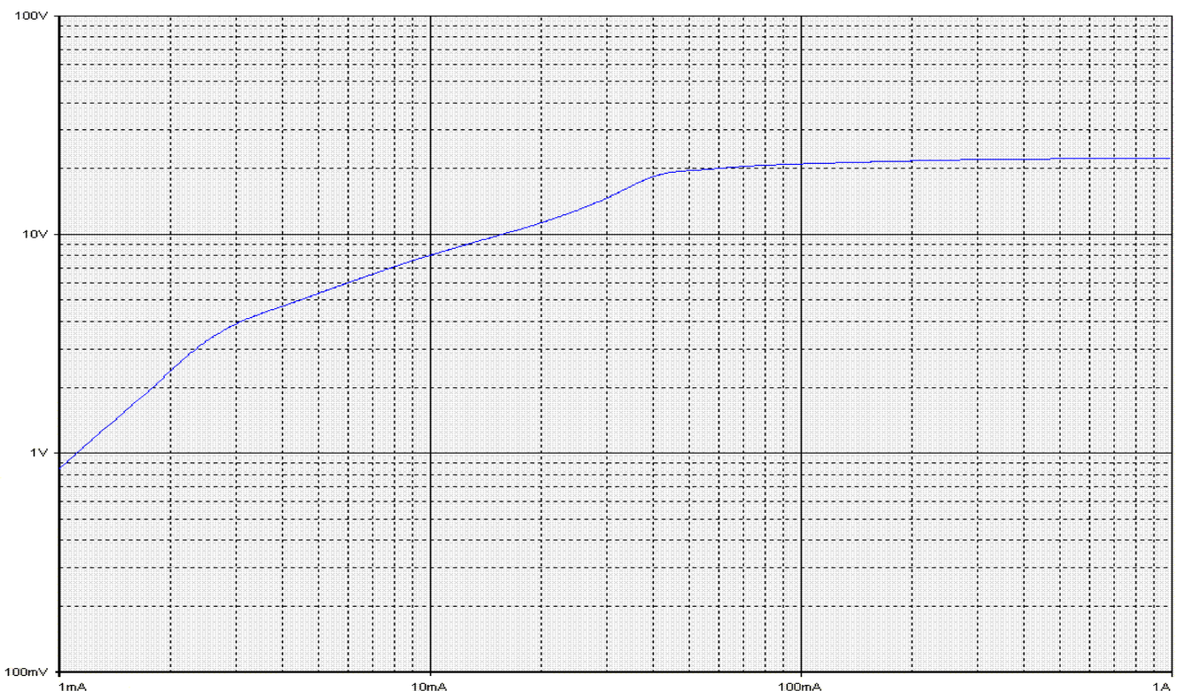
ВАХ вторичной обмотки для измерения с КТ 0,2; 0,2S, номинальной нагрузкой 10 \text{ В} \cdot \text{А} и K_{\text{БНОМ}}=10 трансформаторов с первичным током 1500 А. Сопротивление обмотки постоянному току – 0,18 Ом.
