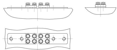
Рис. 3 Остальное см. рис. 1 Трансформатор тока с переключением по первичной стороне
